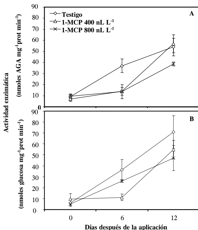
Figura 3. Efecto del 1-MCP sobre la actividad de poligalacturonasa (A) y celulasa (B) en frutos de mango ‘Ataulfo’ almacenados a 20 °C. Los datos son media ± error estándar (n = 4).
