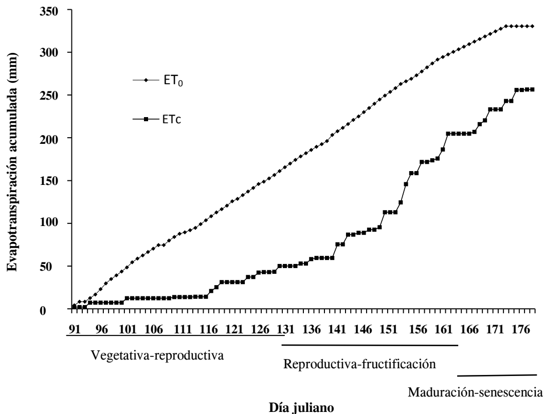
Figura 3. Evapotranspiración acumulada de ET_c y ET_0 en el cultivo de tomate de cáscara sin acolchado plástico y con riego por goteo.
